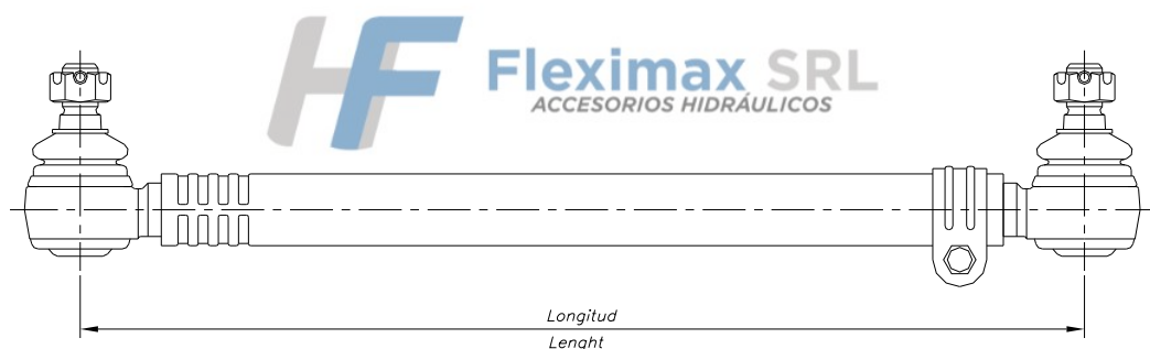
Extremos de dirección Steering tie rod ends
