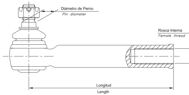
Extremos de direccion Steering Tie Rod Ends
